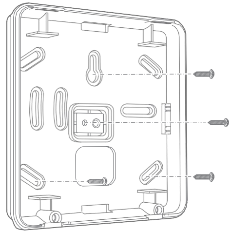
Abbildung 4: Rückwandbefestigung
