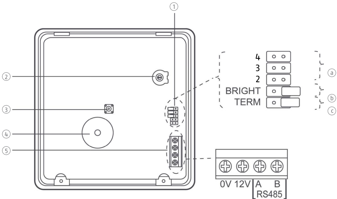
Abbildung 5: Vorderes Kunststoffgehäuse mit Platine
