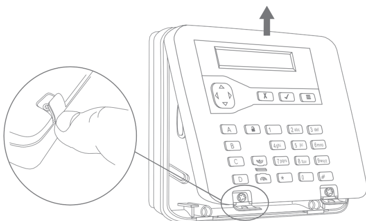
Abbildung 2: Ausbauen der Frontplatte
