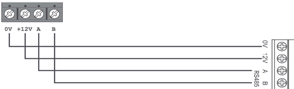
Abbildung 6: Busverkabelung
